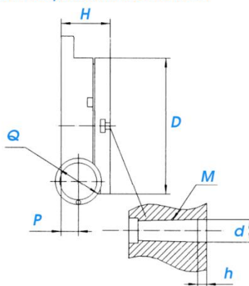
Столы поворотные ТИП 5030 TS..A
