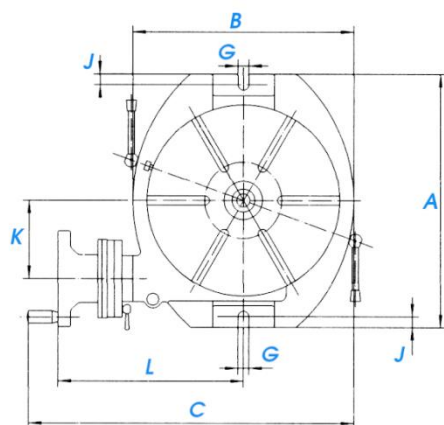
Столы поворотные ТИП 5030 TS..A
